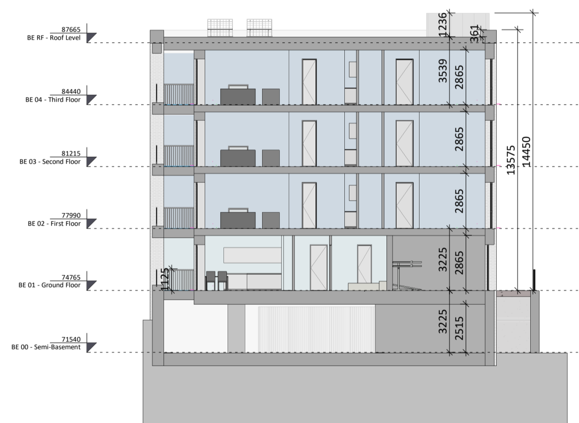
5 BE - Section AA 1 : 200
